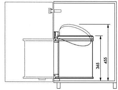
Detailansicht: Einbaumaße
