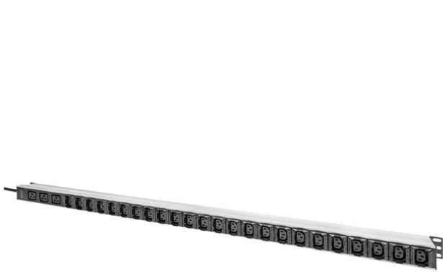
19" Kaltgeräte-Steckdosenleiste, 27-fach
