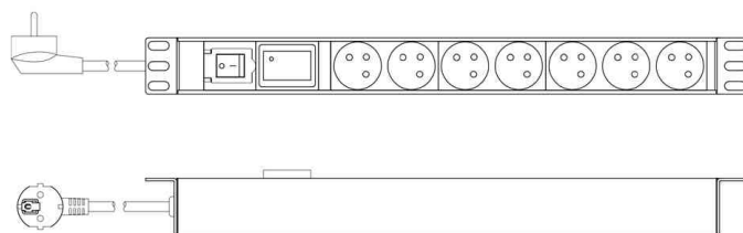
Visuel de référence : multiprise 19" avec interrupteur
