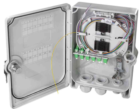
FTTH / FTTB-Anschlussgehäuse, bestückt
