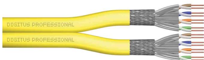
Twisted Pair Installationskabel Kat. 7A, Duplex
