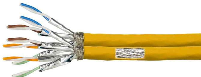
Symbolbild: Installationskabel Kat. 7A, S/FTP - 1.200 MHz, Duplex
