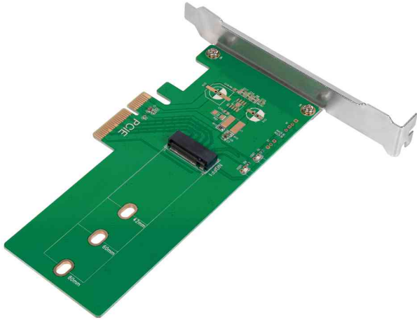
PCIe - M.2 PCI-Express Karte SSD
