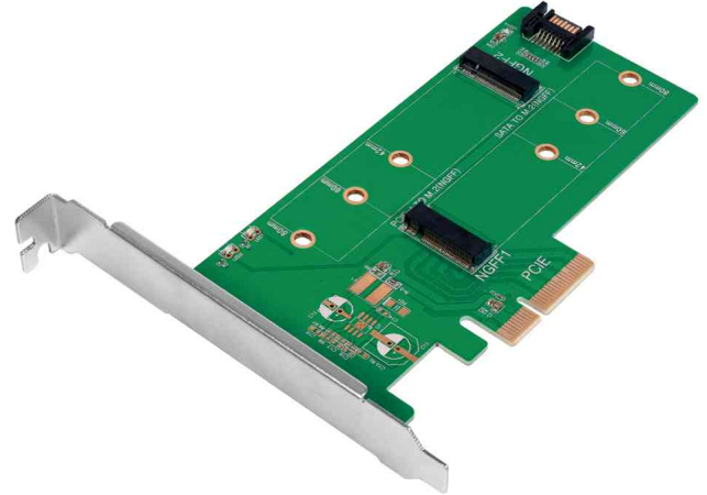
Dual M.2 PCI-Express Karte für SATA & PCIe SATA SSD
