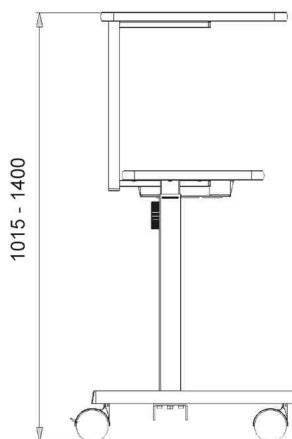
Projektionswagen EuroLine DVP II, Skizze
