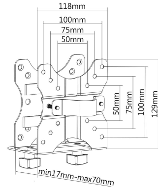
Mini Desktop PC-Halter, Maße
