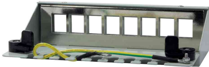
Stahlgehäuse für 8 Keystone Module
