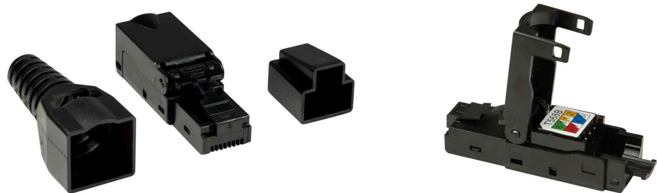
RJ45-Steckverbinder EconLine Kat.6A, T568A, ungeschirmt
