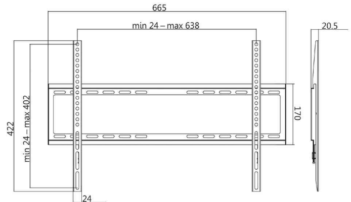
TV-Wandhalterung - Abmessungen
