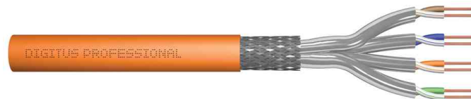
Installationskabel Kat. 7, S/FTP, PiMF, duplex
