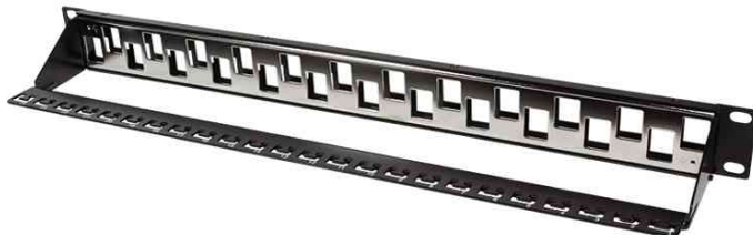
19" Keystone Patch Panel, 24 Port, schwarz, Rückseite
