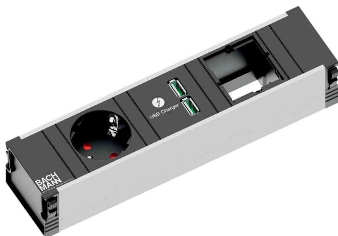
Steckdoseneinheit CONI
