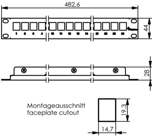
Strichzeichnung
