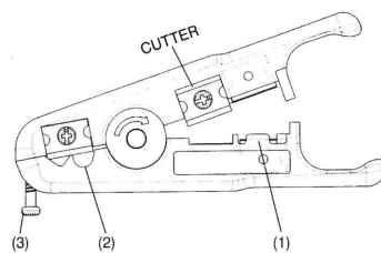
Abisolierwerkzeug
