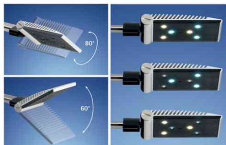
Leuchtenkopf 60° neigbar / 80° schwenkbar - Warmweiße und kaltweiße LED's getrennt dimmbar
