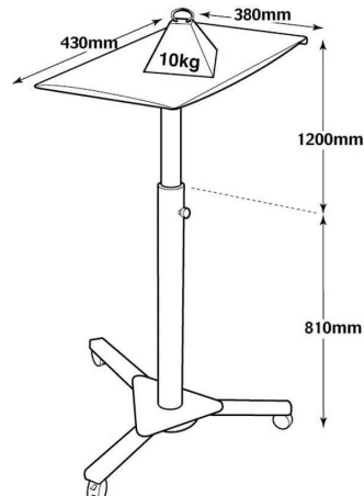
DV- / Dia-Projektionswagen, mit Maßangaben
