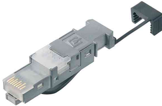
STX RJ45 Stecker AWG 22 - 26, mit schwarzem Farbkodierring
