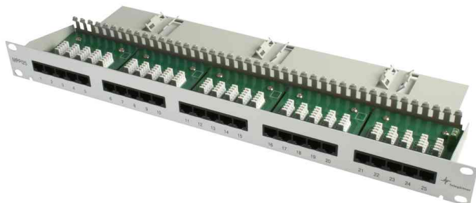
19" ISDN Patch Panel mit Adermanagement
