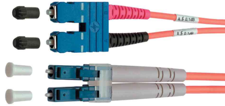
Symbolbild! LWL Patchkabel, LC-Duplex Stecker - SC-Duplex Stecker, OM2
